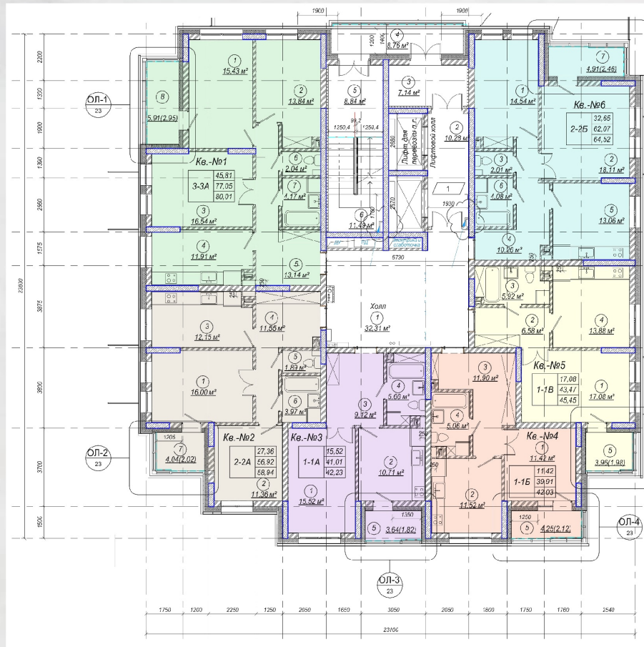
План 2 этажа дома 1.1
